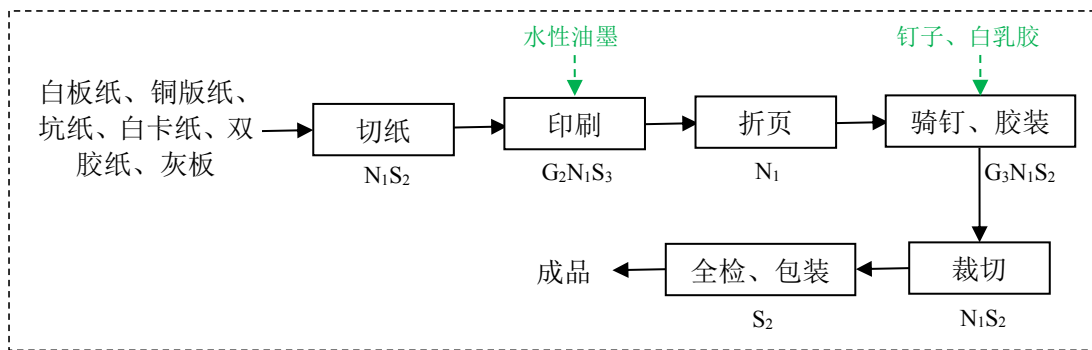
图 2-2 出版物印刷、设计制作印刷品广告生产工艺流程图
