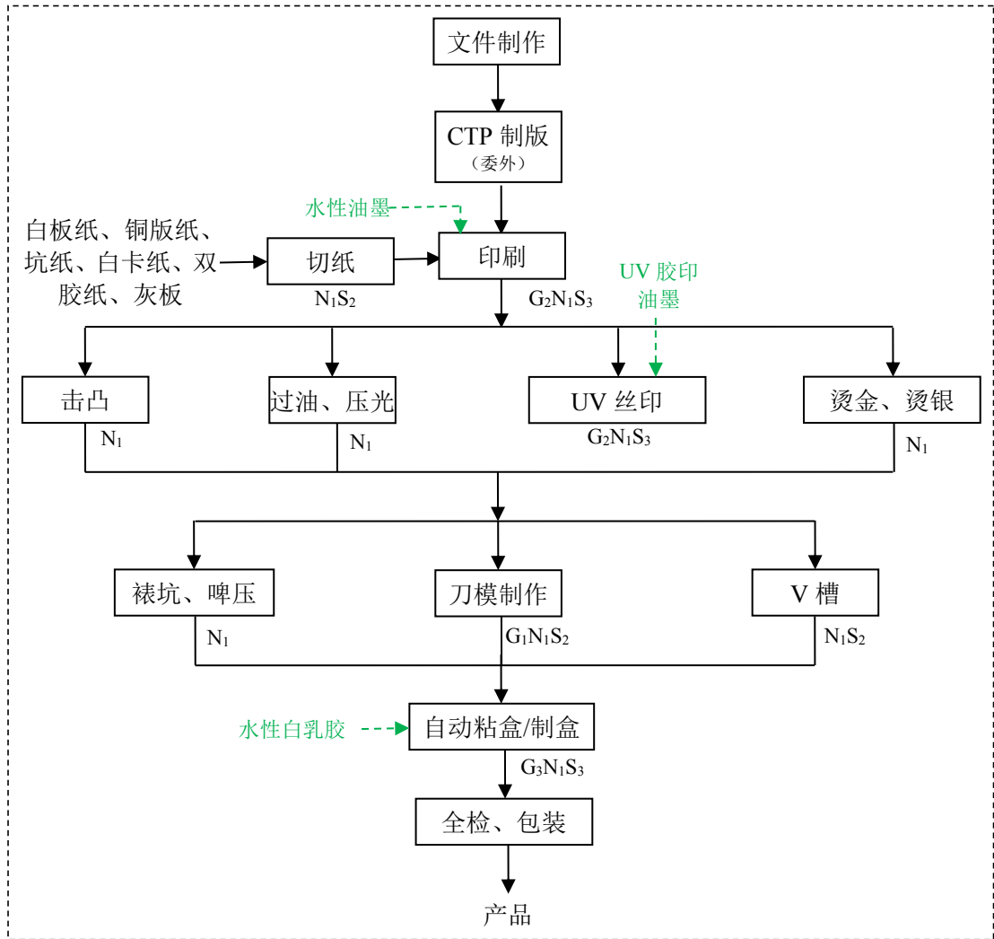
图 2-1 包装装潢印刷品印刷生产工艺流程图
