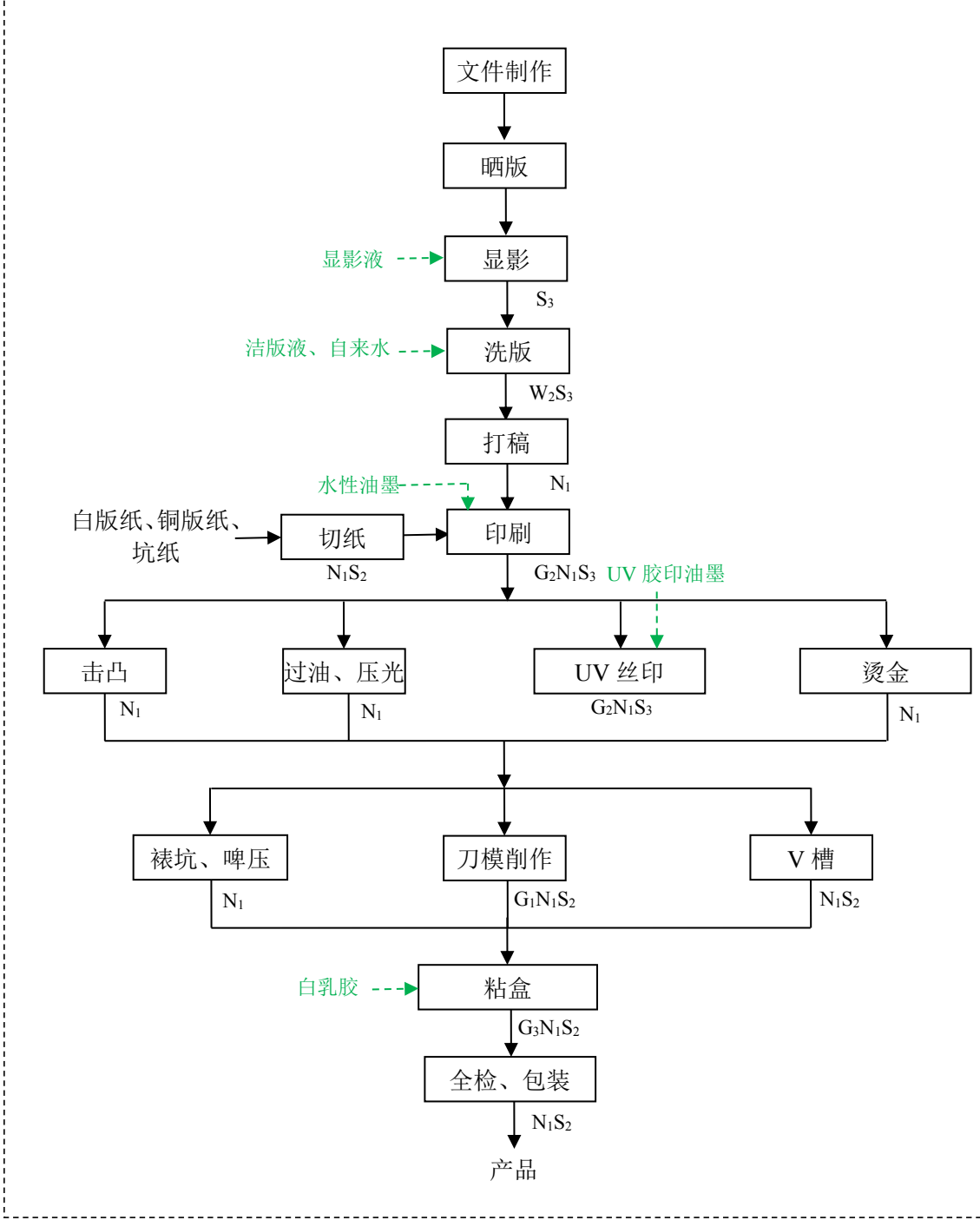
图 2-3 原项目包装装潢印刷品印刷生产工艺流程图
