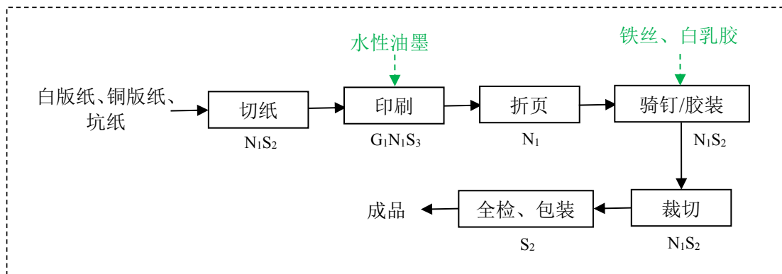
图 2-4 原项目出版物印刷、设计制作印刷品广告生产工艺流程图
