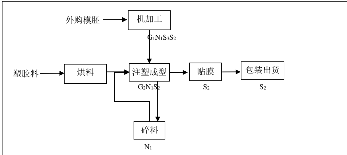
图 2-1 项目生产工艺流程图
