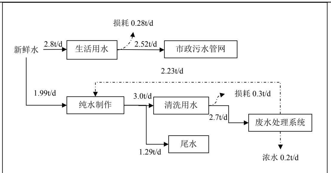
图 4-2 项目全厂水平衡图
