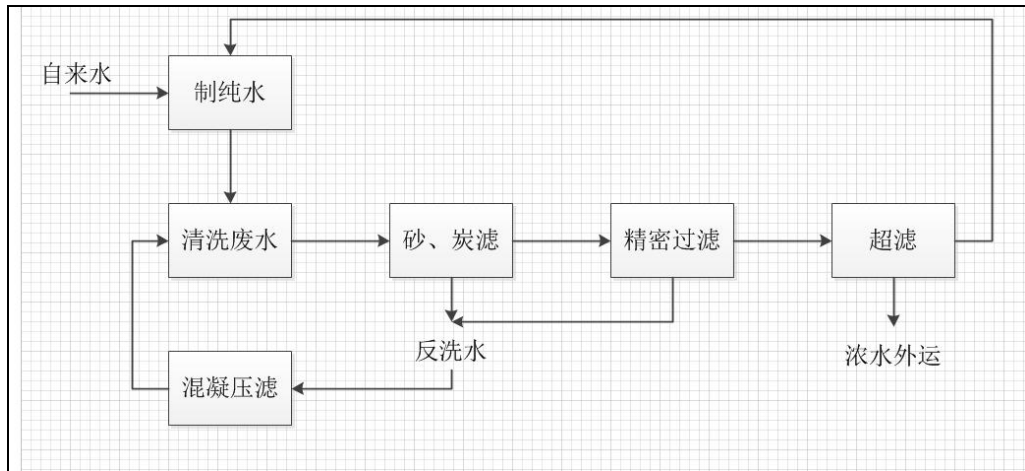
图 4-1 项目废水处理流程图
