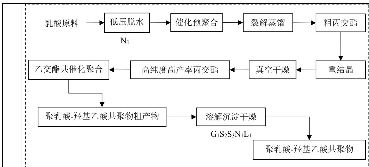
图 2-4 项目聚乳酸-羟基乙酸共聚物研发工艺流程图
