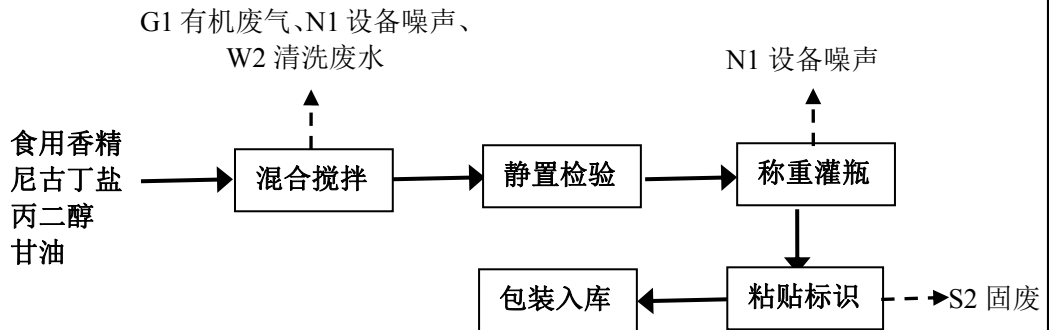
图 2 项目生产工艺流程图
