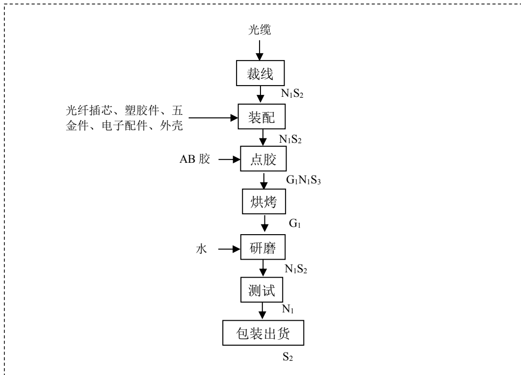
图 2-2 原项目生产工艺流程图
