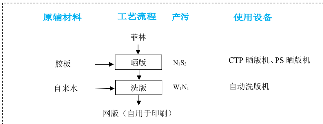
图 2-4 项目丝印、印刷所用网版的晒版工艺流程图
