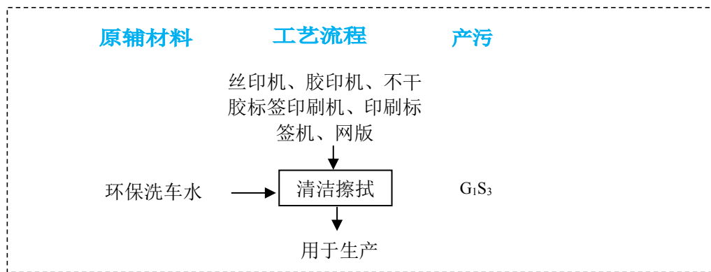
图 2-5 项目设备清洁流程图
