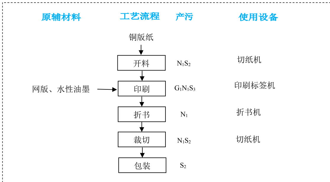
图 2-3 项目纸制品的加工、其他印刷品印刷工艺流程图
