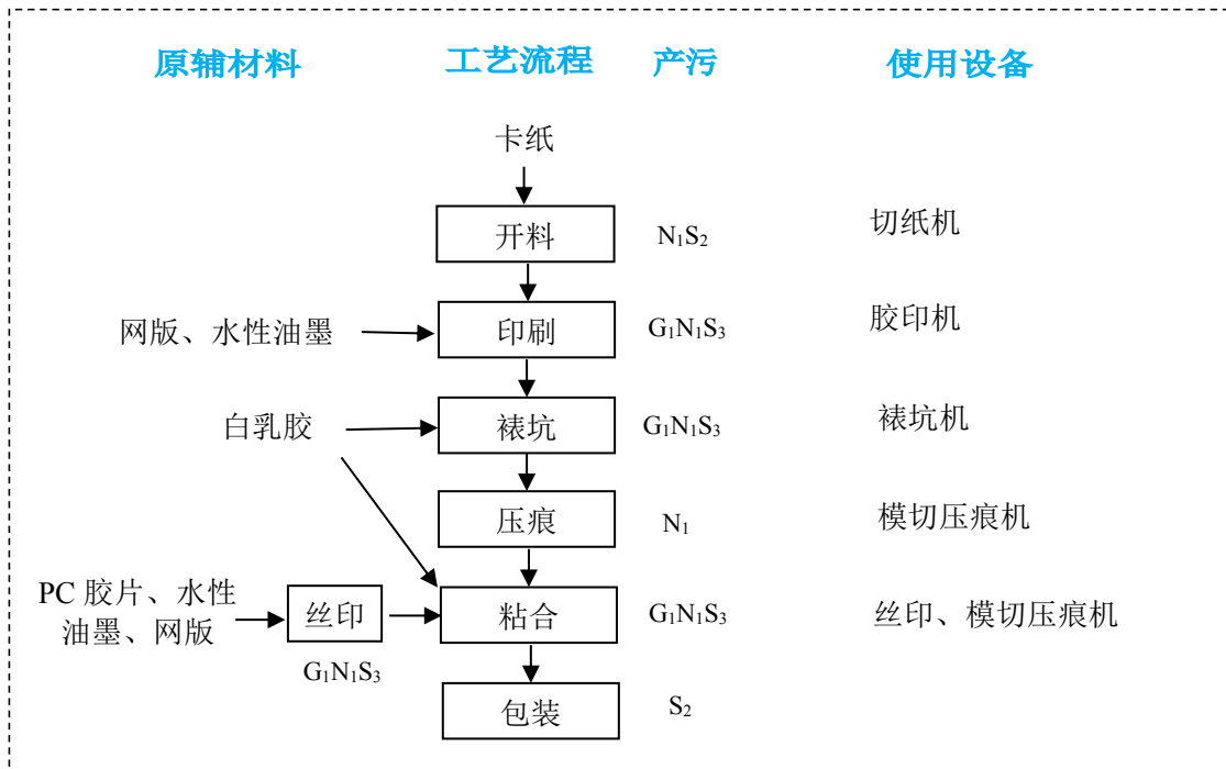
图 2-2 项目包装装潢印刷品生产工艺流程图
