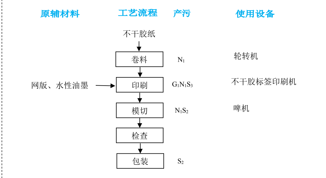
图 2-1 项目不干胶标签贴纸生产工艺流程图
