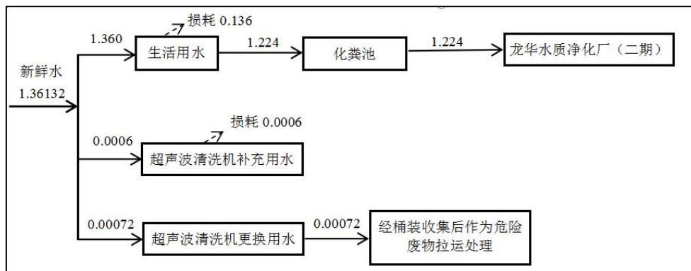
图 4-1 项目水平衡图 单位：t/d
