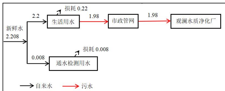
图 4-1 项目水平衡图 单位：t/d
